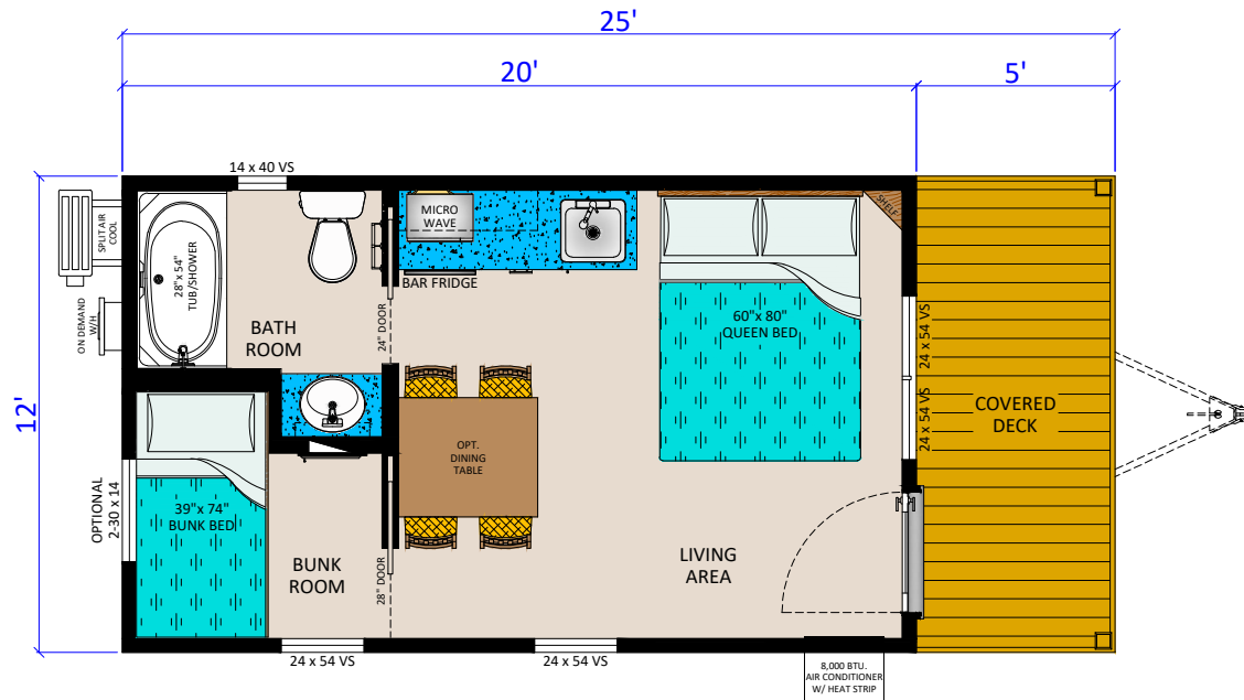
CABANA 21/KOA - 25FP (240 SQ.FT.)+(DECK)
