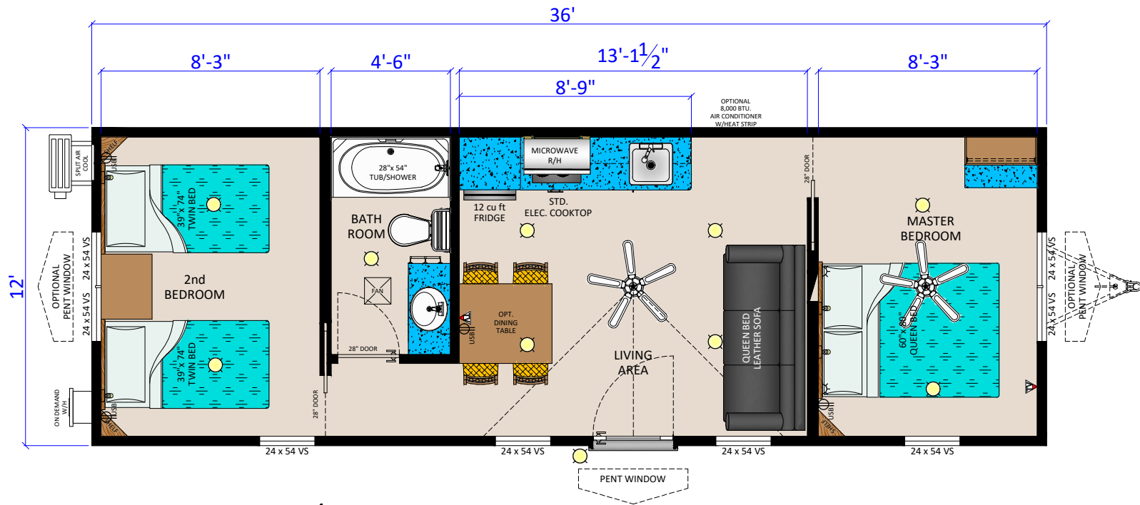
CHILLIWACK 20/KOA - 36S (432 SQ.FT.)
